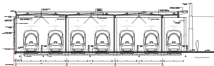
coupe espace de remisage
